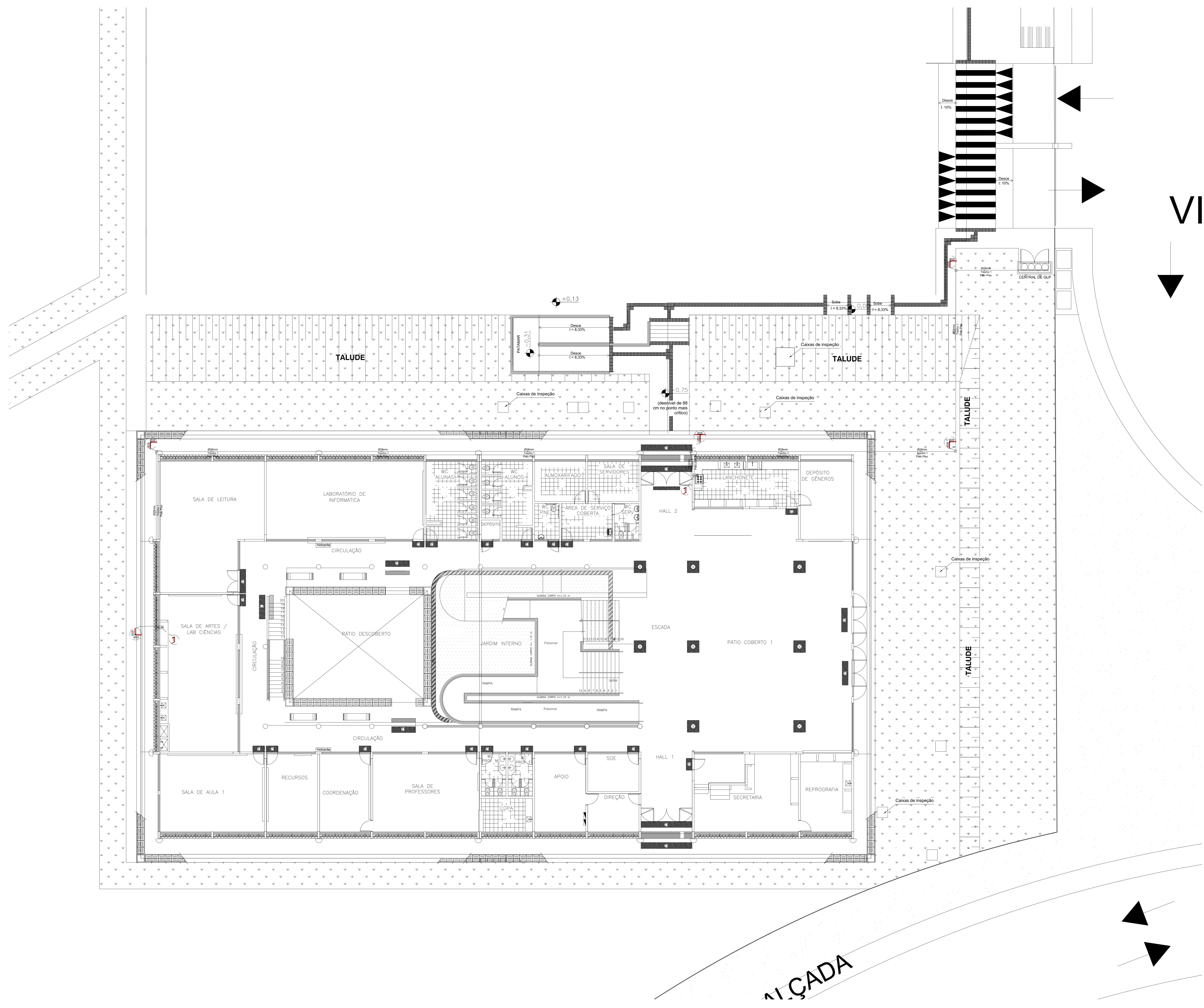
PLANTA GÁS 1 : 100
